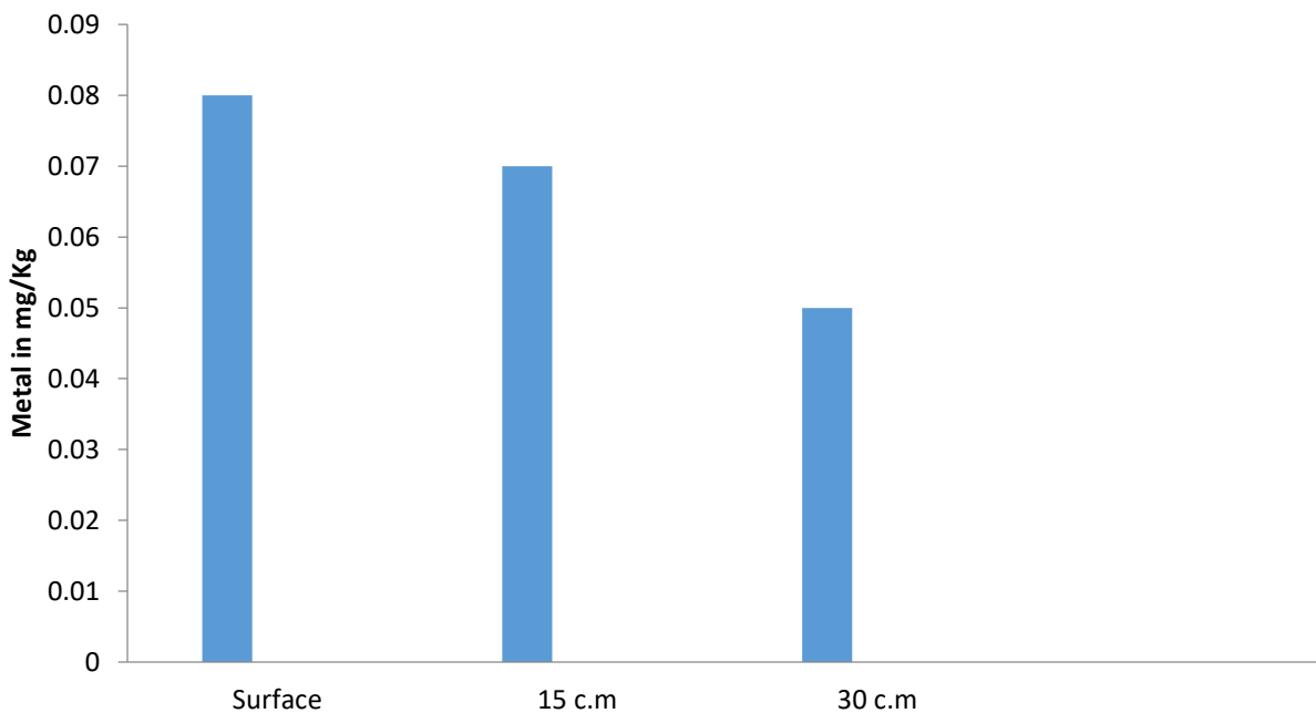
Fig:3 Cadmium(Cd)
